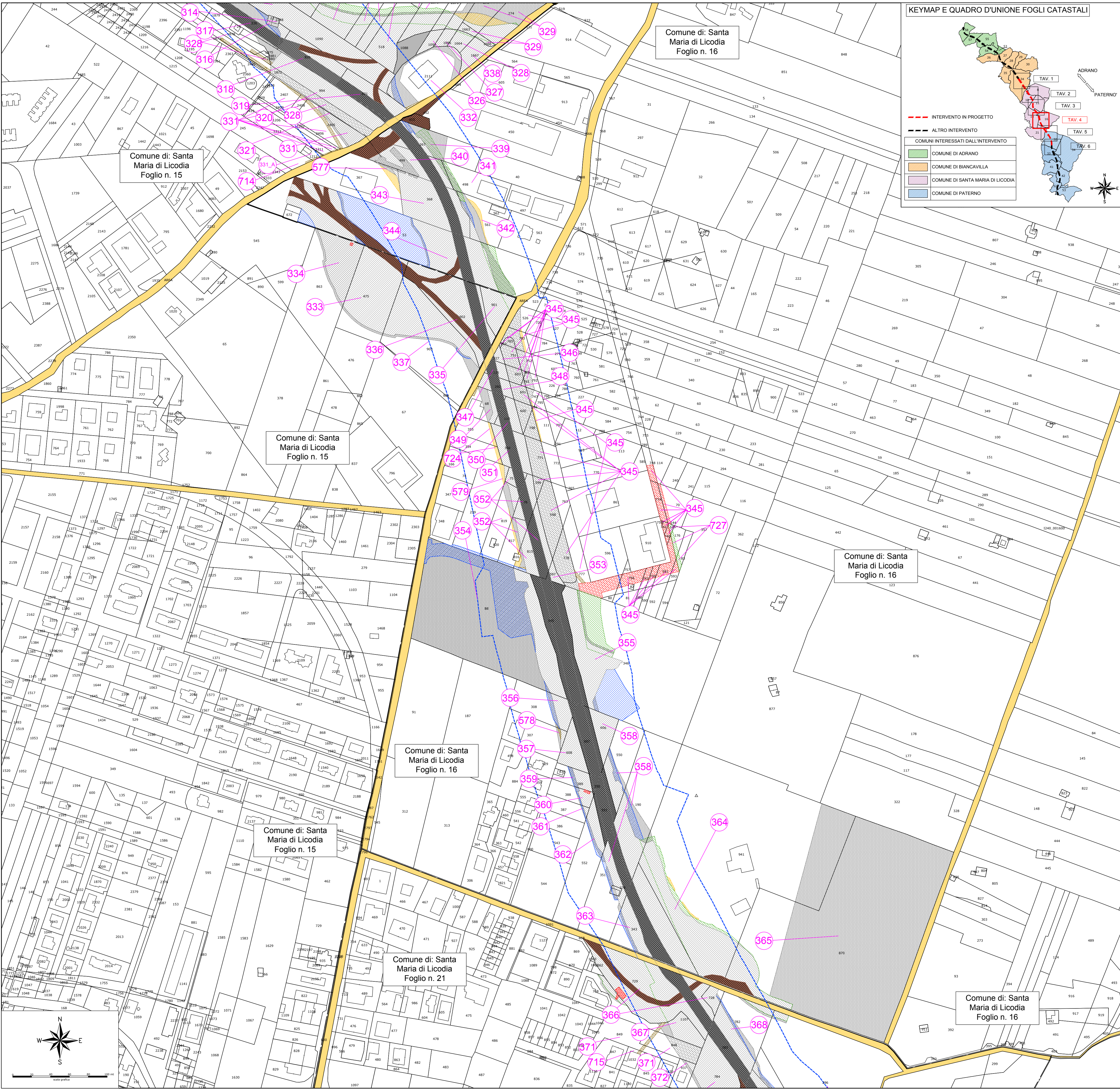
KEYMAP E QUADRO D'UNIONE FOGLI CATASTALI
