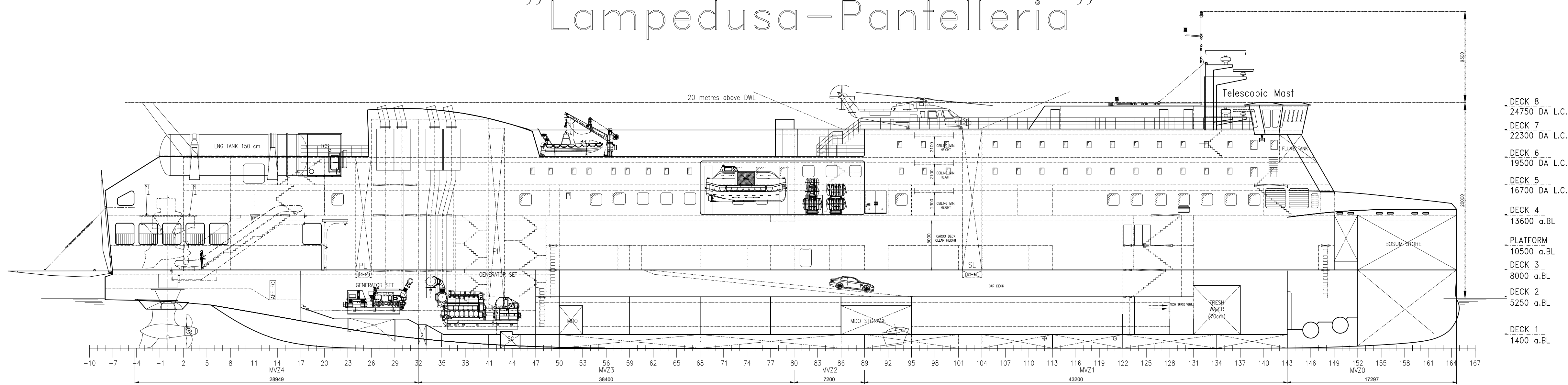
DECK 7 22300 DA L.C.
