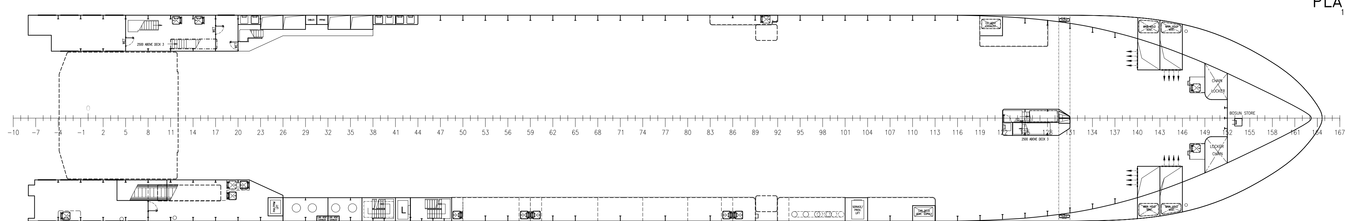
PLATFORM 10500 DA L.C.
