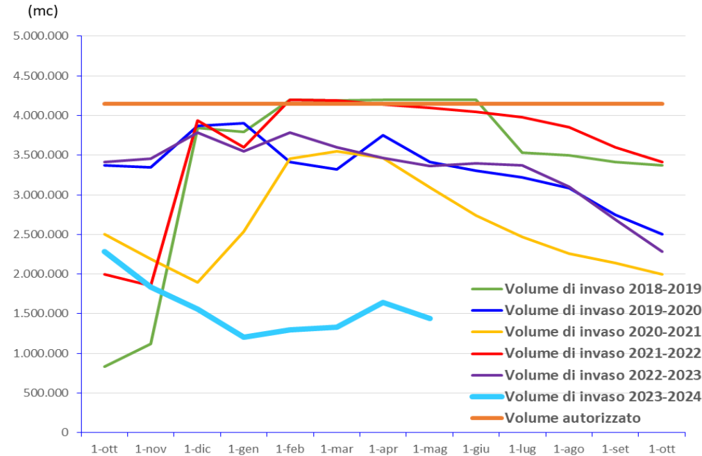
Diga Ogliastro (Don Sturzo) - Ente Gestore: C.B. Sicilia Or. Andamento volume totale di invaso (mc) Anno idrologico (1 ott - 30 set)
