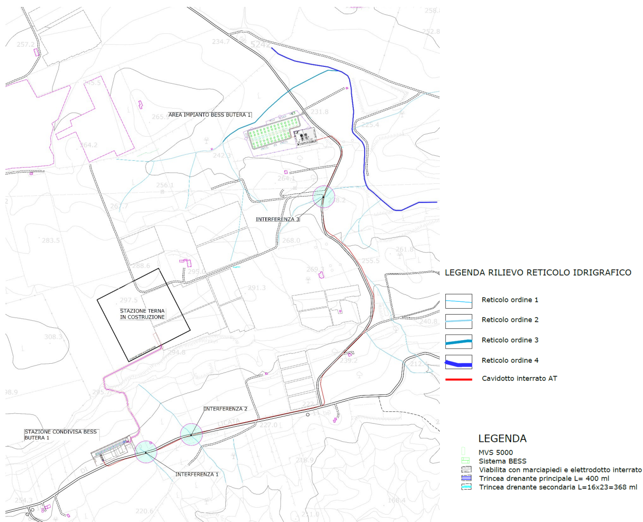
Figura 1 Planimetria Intervento
